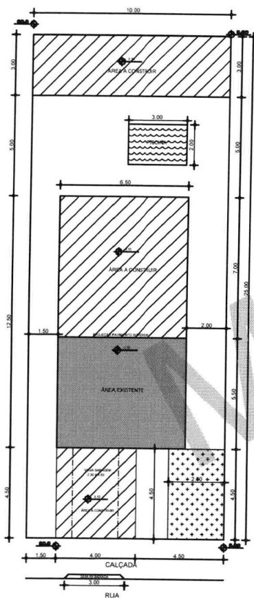
PAVIMENTO TÉRREO ESC: 1:100
